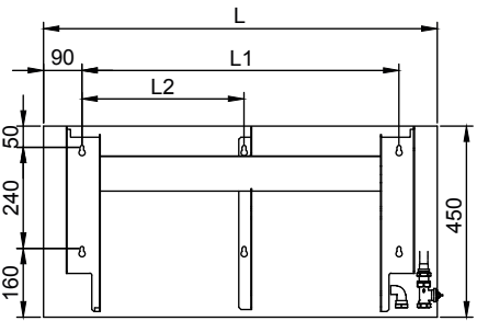
KORAWALL WK xxx/60/6-12
